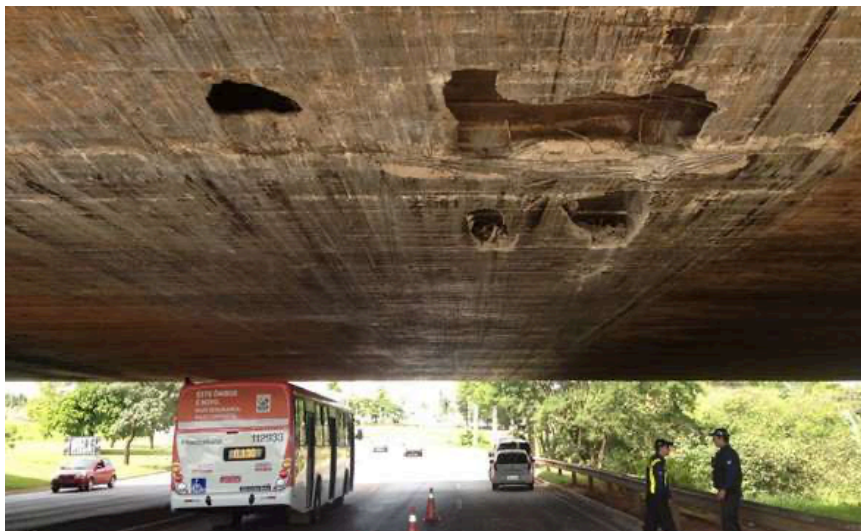
Figura 12: Danos na laje inferior do caixão perdido
