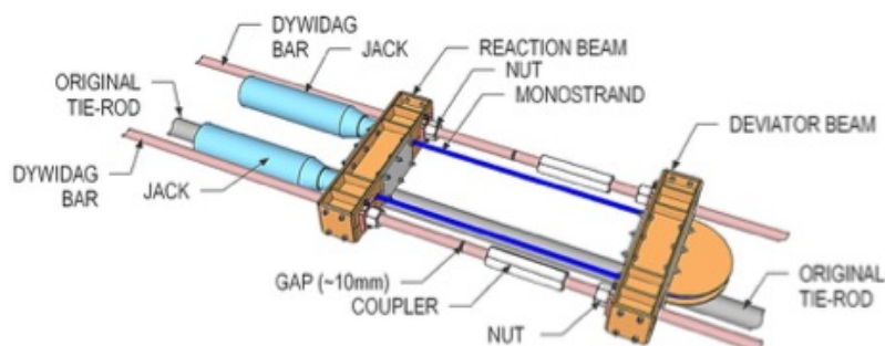
FIGURA 24: TENSIONAMENTO INDIRETO DAS BARRAS
