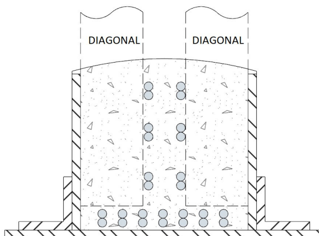
FIGURA 22: INCORPORAÇÃO DE VERGALHÕES
