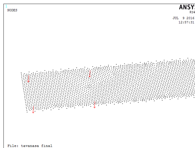
FIGURA 16: APLICAÇÃO DE CARGAS PONTUAIS AOS NÓS DO TABULEIRO EQUIVALENTE AO TREM TIPO DE 120 KN
