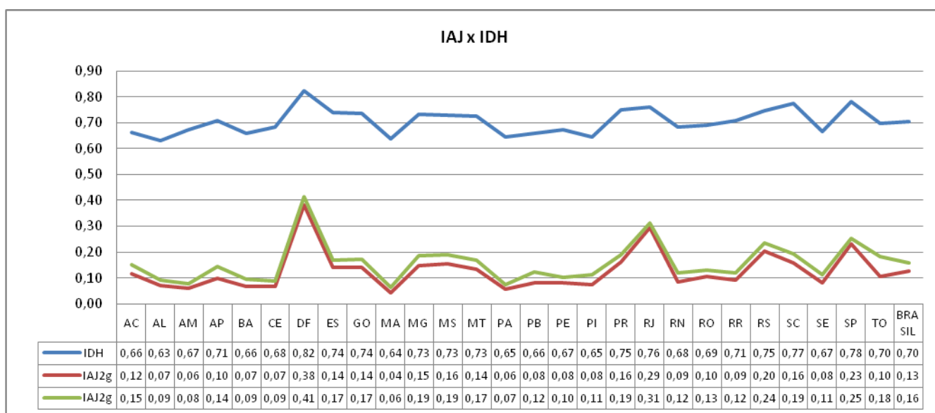
Gráf.21 – IAJ-IDH, comparação IAJ x IDH, visão tradicional do SJ somente com Judiciário, MP e advocacia.
