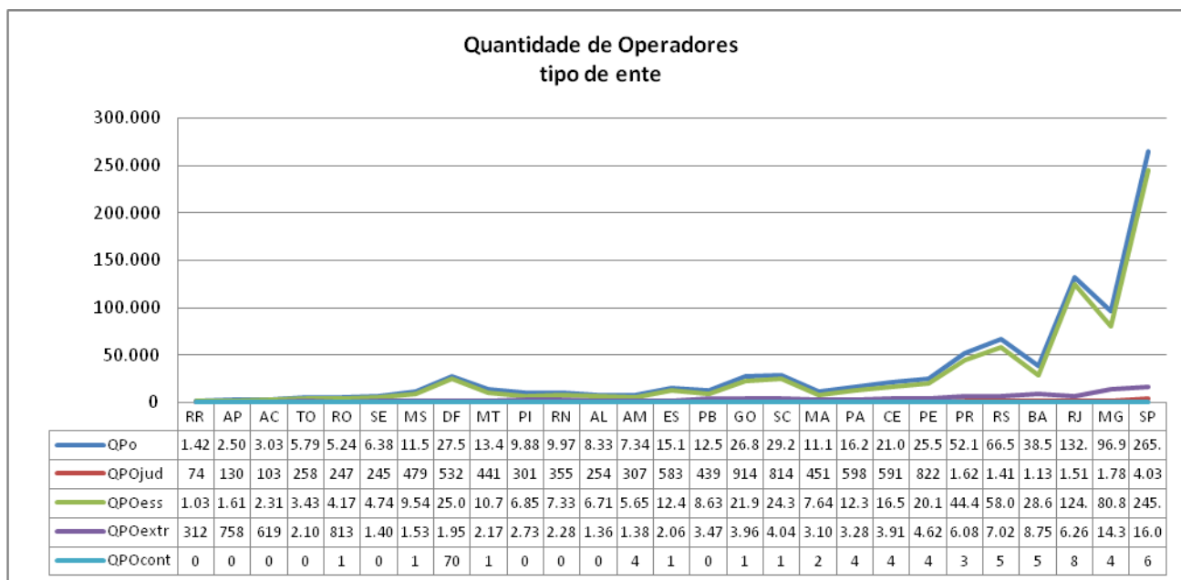
Gráf.3 - Quantidade de Operadores SJ, ordenado por população
