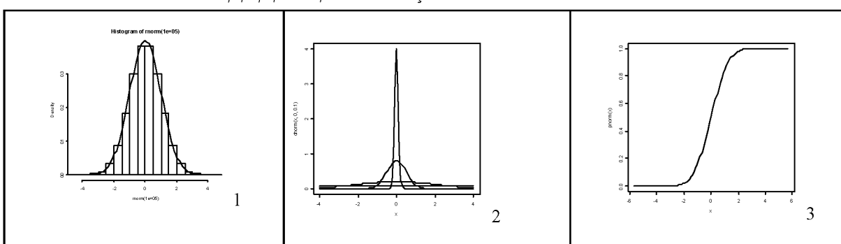
GRÁFICOS 1,2 E 3 - DENSIDADE DE PROB. NORMAL PADRÃO [0,1]; DIFERENTES NORMAIS COM VARIÂNCIAS: 0,1; 0,5; 2 E 4;. DISTRIBUIÇÃO DE PROBABILIDADES NORMAL
