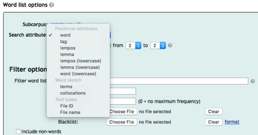
Figura 7: Criação de wordlist com opções de base. Fonte: Autora
