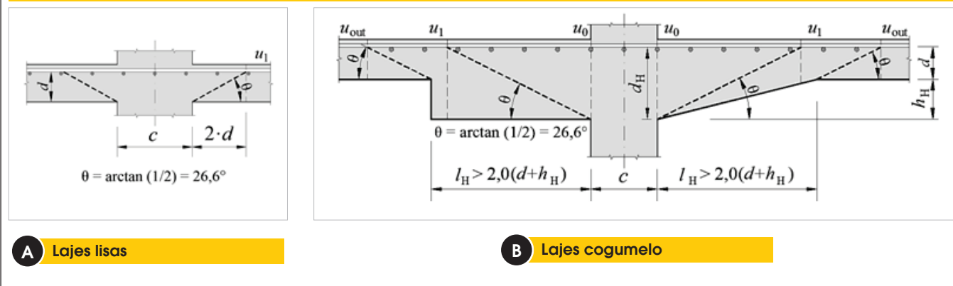
Figura 5 – Modelo de verificação de punção no estado limite último (EUROCODE 2 (11))
