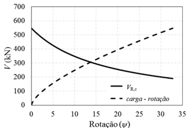
Figura 7 – Representação gráfica do cálculo da carga de ruptura por punção segundo TFCC
