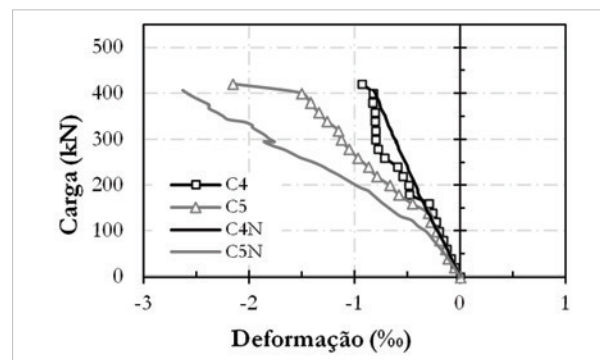
D Deformações radiais na laje LC2
