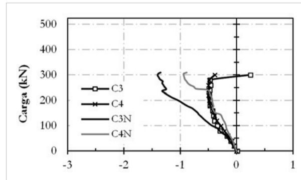
B Deformações radiais na laje LC1
