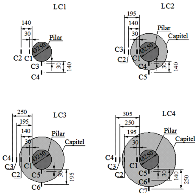
Figura 9 – Extensômetros fixados no concreto na face inferior das lajes
