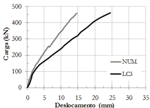
C Deslocamentos da laje LC3
