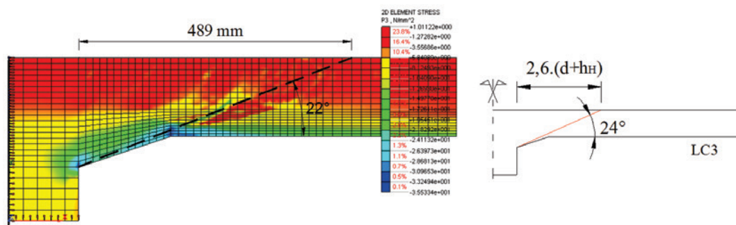
C Tensões de \sigma_{Máx} referente à carga de ruptura do modelo LC3 e o ângulo da superfície de ruína experimental
