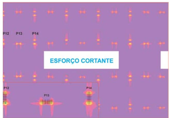
Figura 6 - Contorno dos esforços cortantes nas lajes.
