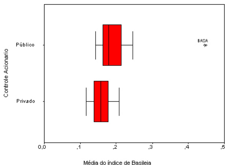
Gráfico 4 – Boxplot do valor médio do Índice de Basileia pelo controle acionário – entre 2001 e 2006
