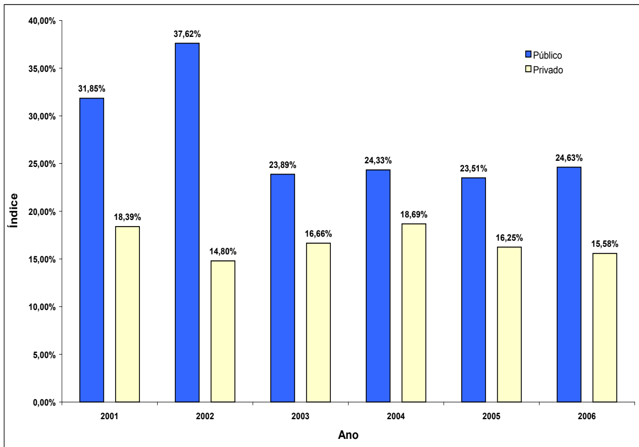
Gráfico 1 – Valor Médio de índice de Basileia por controle acionário – entre 2001 e 2006
