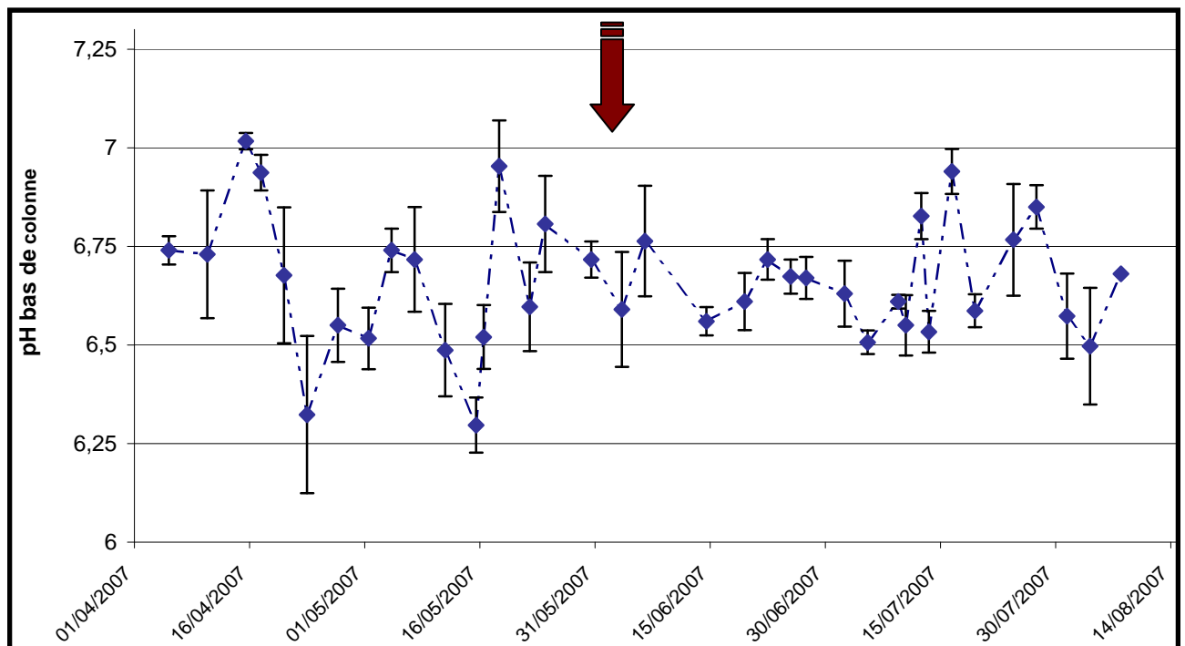
Figure V_6 – Evolution du pH moyen des eaux de percolation au cours du temps, (↓ ajout de MO).
