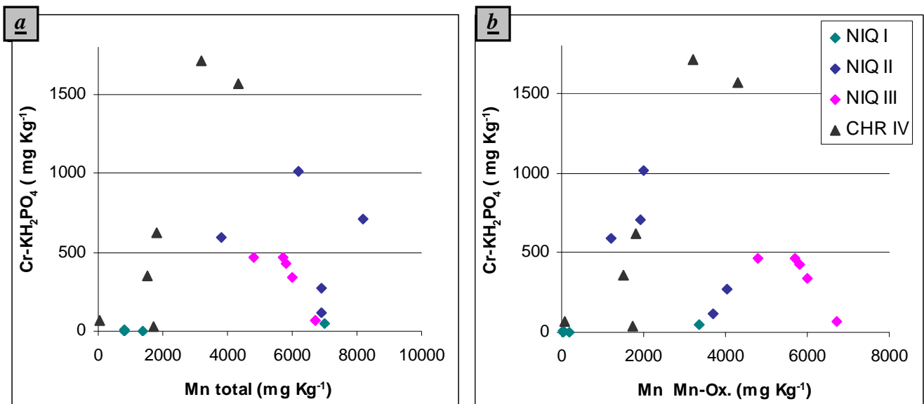
Figure V_13 – Relation entre le Cr(VI) disponible et la teneur en Mn a) et en oxydes de Mn b) des sols.
