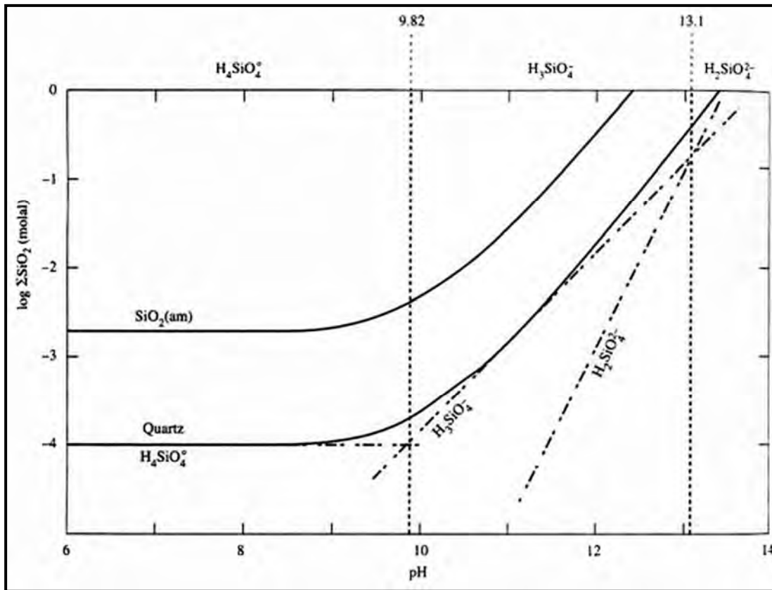
Figure V_7 – Diagramme de stabilité de la silice à 20°C.
