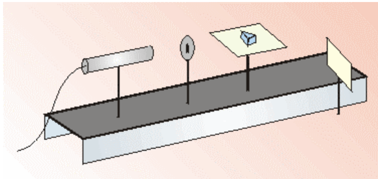
Figura 17: montagem experimental
