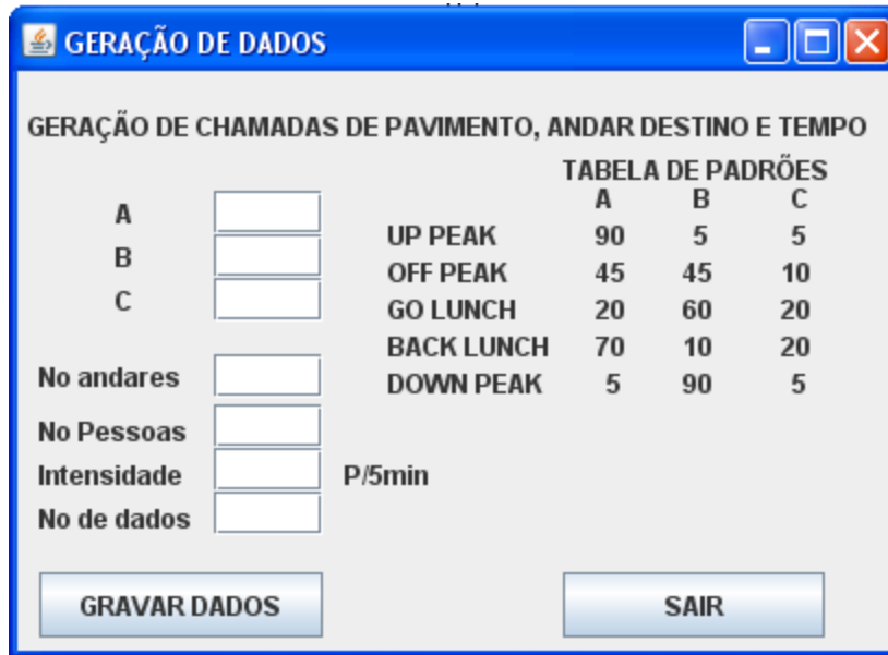
Figura 3-3- Interface gráfica para geração de tráfego de chamadas (submódulo parâmetros gerador de tráfego)
