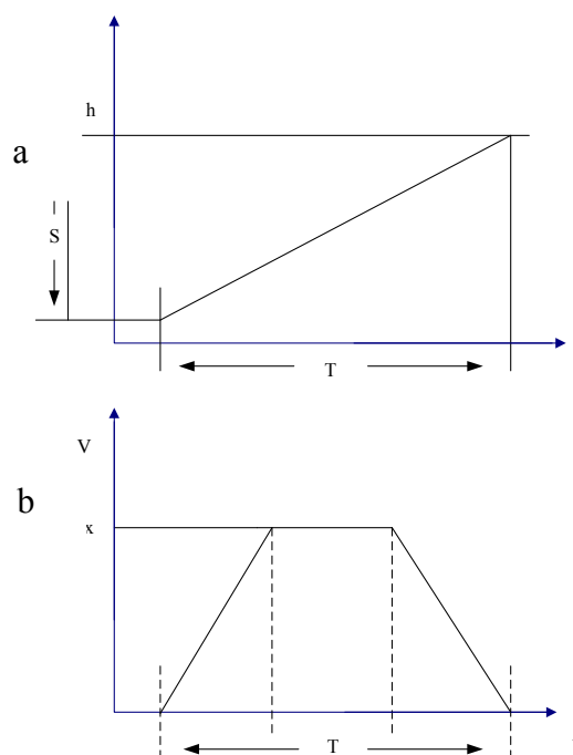
Figura 3-4 — Gráfico (a) representa a distância percorrida por um elevador. Gráfico (b) representa a curva de velocidade ( v_{\max} ) de um elevador entre duas paradas em andares subsequentes
