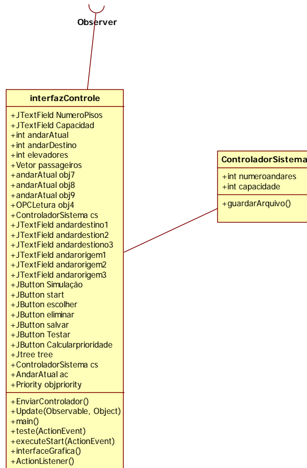
Figura 4-15 – Diagrama de classes de configurar controle
