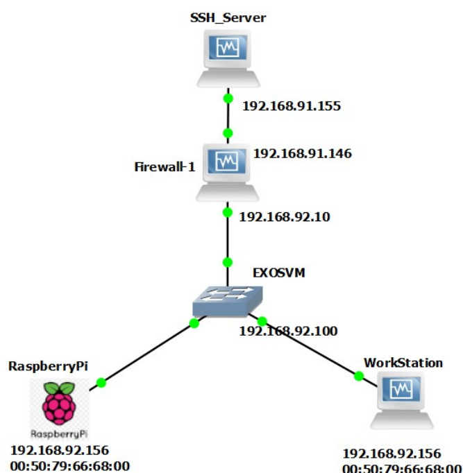
Figura 4.4: Arquitetura do laboratório para Teste de Bloqueio de Tráfego
