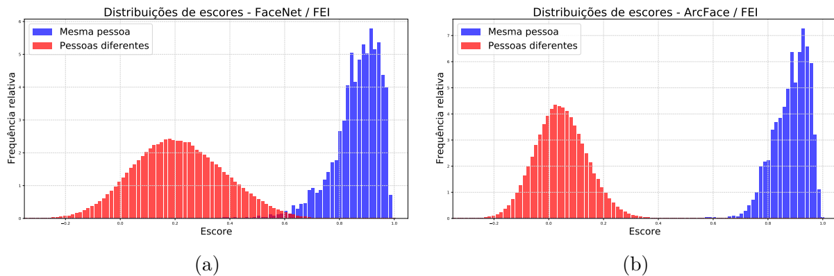
Figura 4.2: Distribuições de escores na base FEI obtidas com o FaceNet (à esquerda) e com o ArcFace (à direita).
