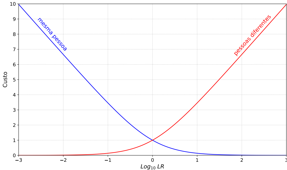
Figura 4.11: Funções de custo que compõem a C_{lr} . Adaptada de [13].
