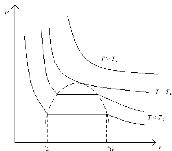
Figura 2 - Isotermas nas vizinhanças de um ponto crítico
