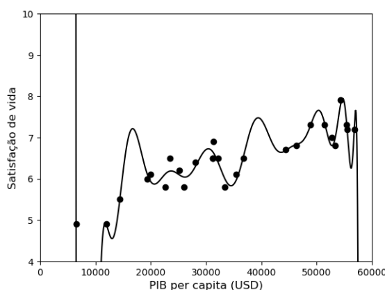
Figura 3 – Modelo com sobreajuste nos dados de treinamento
