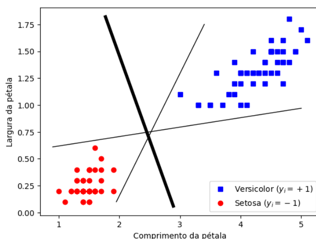
Figura 10 – Três hiperplanos, mas somente um tem maior margem de separação
