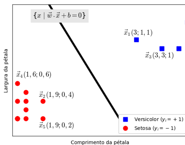
Figura 18 – Exercício da flor íris para discentes
