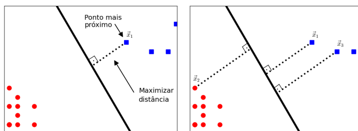
Figura 17 – Resumo esquemático usando abordagem com rigor intermediário
