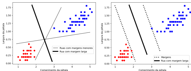
Figura 16 – Resumo esquemático usando abordagem lúdica
