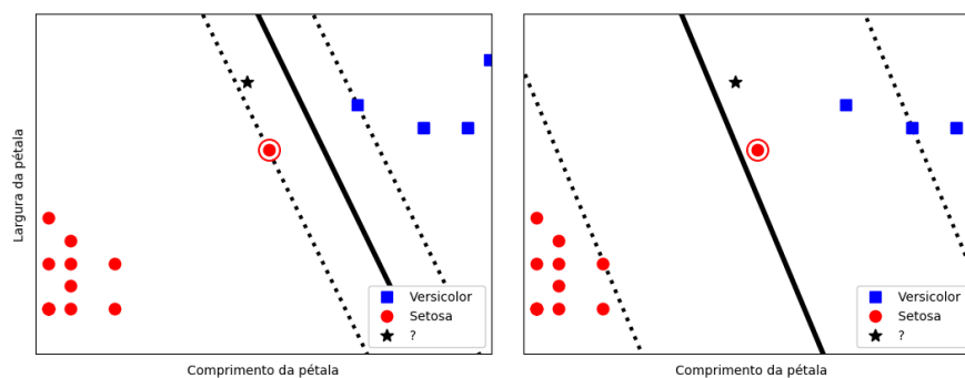
Figura 14 – Margem rígida (à esquerda) e margem que permite violações (à direita)
