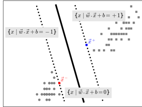
Figura 13 – Hiperplano com destaque dos vetores de suporte e margens
