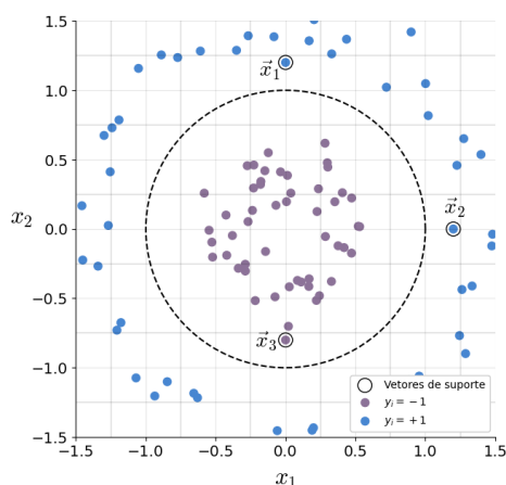
Figura 22 – Resumo esquemático segunda atividade I e II
