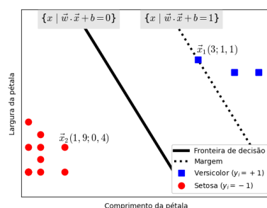
Figura 20 – Resumo esquemático primeira atividade II
