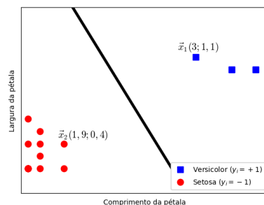
Figura 19 – Resumo esquemático primeira atividade I
