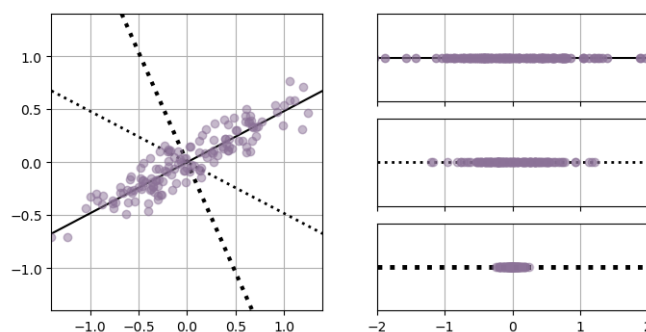
Figura 8 – Três possíveis retas para projeção dos dados
