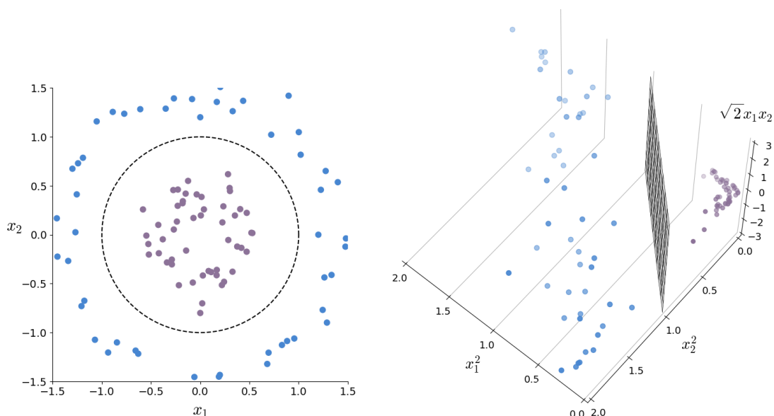
Figura 15 – Ilustração didática do truque do kernel
