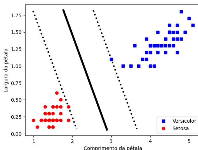
Figura 11 – Hiperplano de margem larga com vetores de suporte nas margens
