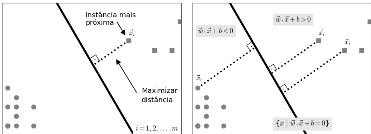
Figura 12 – Hiperplano que maximiza sua distância até as instâncias mais próximas
