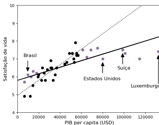
Figura 9 – Regressão linear nos dados completos
