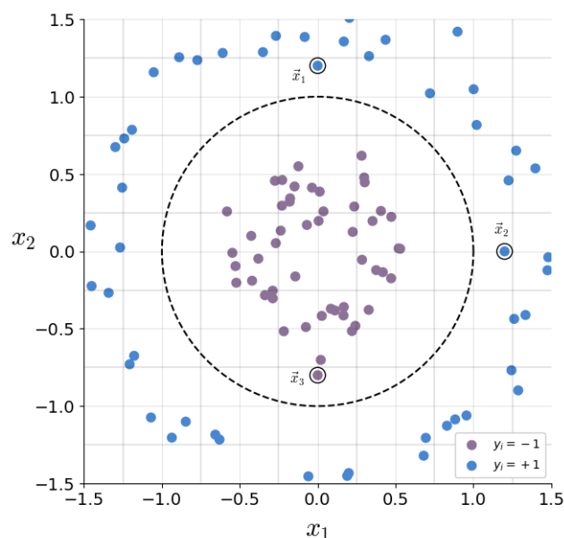
Figura 21 – Exercício com o truque do kernel para discentes
