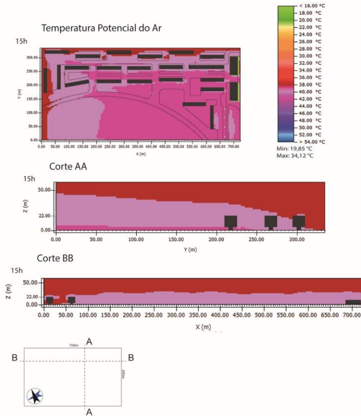
Figura 05 - Simulação Computacional - ENVI MET - 15 horas (Elaboração Própria – plugin LEONARDO, Envi-Met v.4.4.3).
