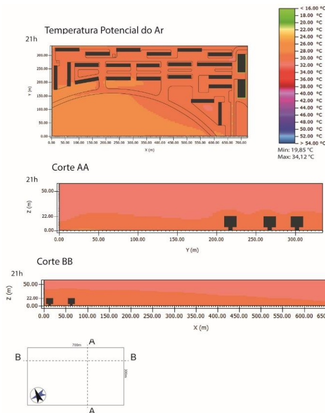
Figura 06 - Simulação Computacional - ENVI MET - 21 horas. (Elaboração Própria – plugin LEONARDO, Envi-Met v.4.4.3)
