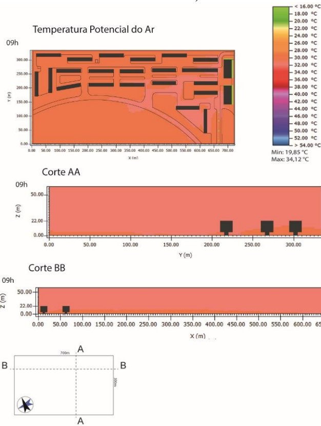
Figura 04 - Simulação Computacional - ENVI MET - 09 horas (Elaboração Própria – plugin LEONARDO, Envi-Met
