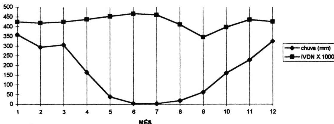
Figura 21- Comparação Gráfica dos Valores Originais Médios Mensais de Chuva e IVDN do GRUPO SETE
