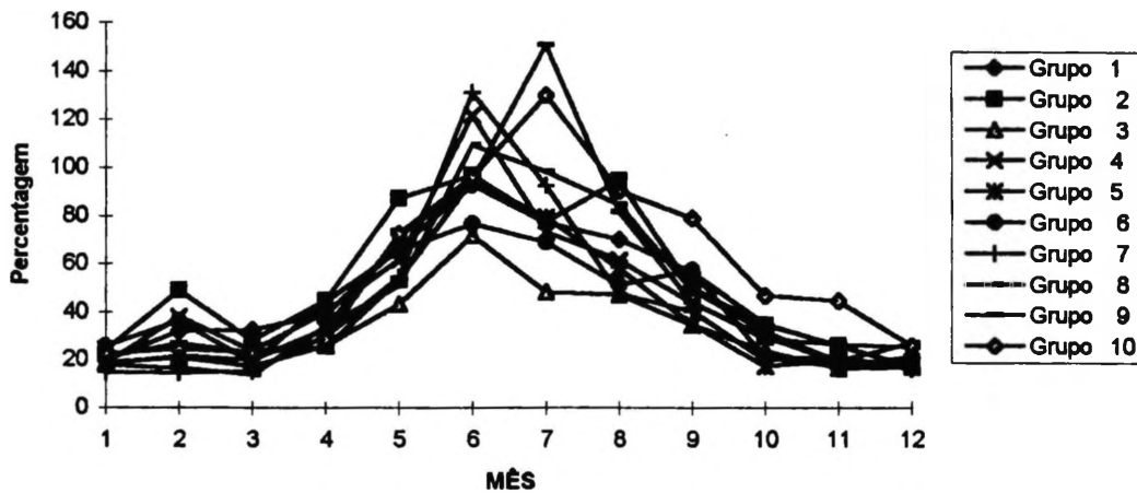
Figura 29- Demonstração Gráfica dos Coeficientes de Variação (%) Mensais da Chuva para os Dez Grupos
