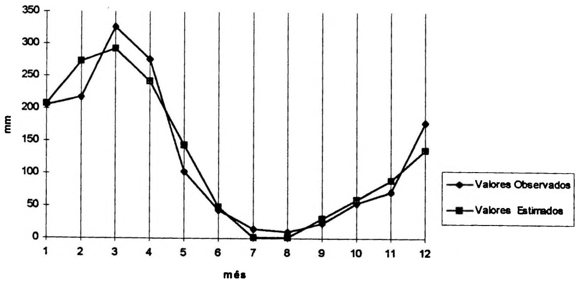
Figura53 Comparação Gráfica dos Valores Observados e Estimados de Chuva para o GRUPO DEZ
