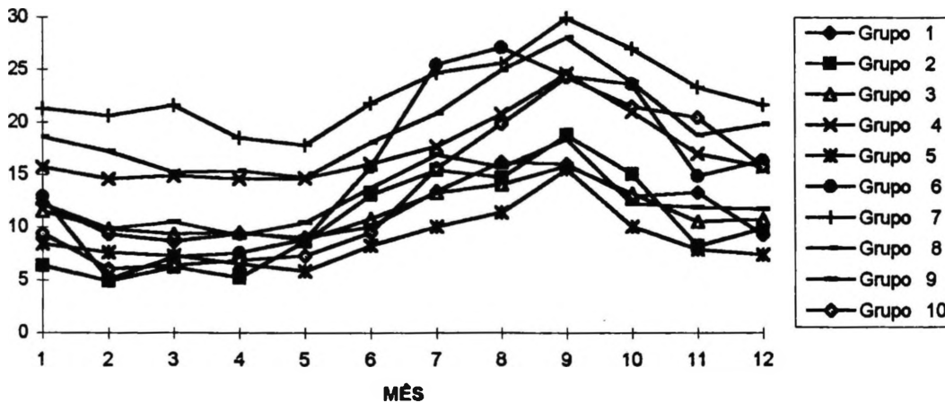
Figura 30- Demonstração Gráfica dos Coeficientes de Variação (%) Mensais dos IVDN para os Dez Grupos
