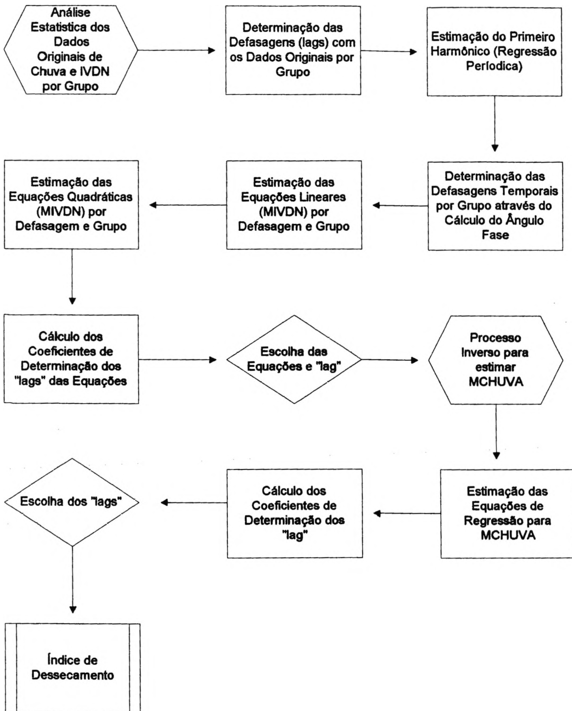
FIGURA 8-FLUXOGRAMA DOS MÉTODOS ESTATÍSTICOS UTILIZADOS PARA O CÁLCULO DO DEFASAMENTO ENTRE CHUVA E IVDN (SEGUNDA FASE)
