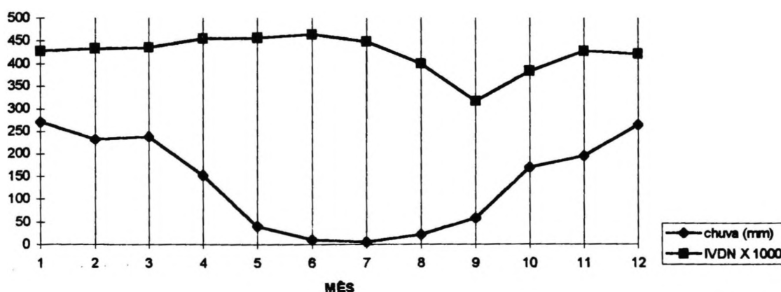
Figura 22- Comparação Gráfica dos Valores Médios Mensais da Chuva e IVDN para o GRUPO OITO
