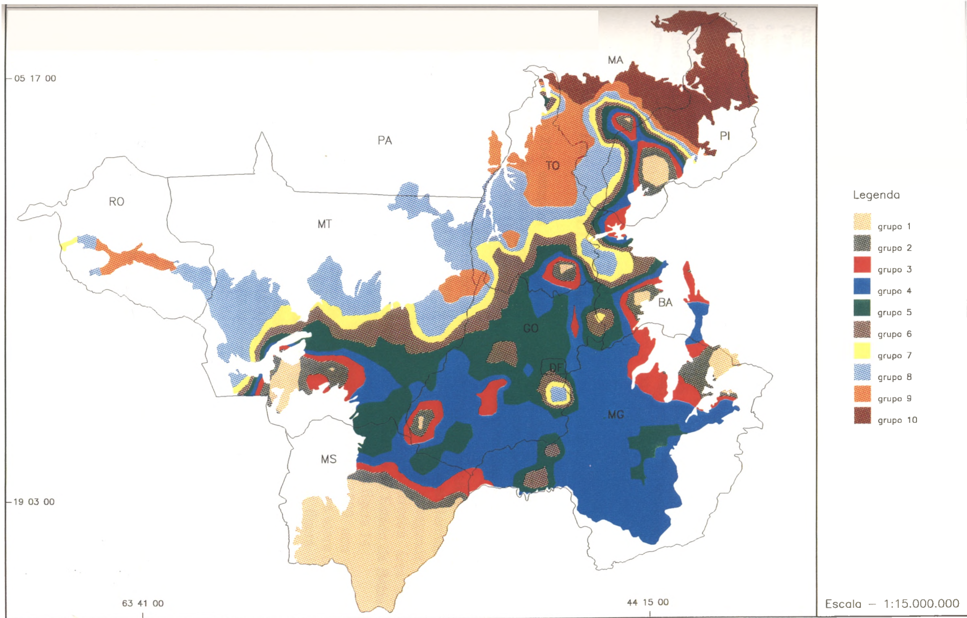
FIGURA 14 DISTRIBUIÇÃO DOS DEZ GRUPOS HOMOGÊNEOS DENTRO DO BIOMA DO CERRADO
