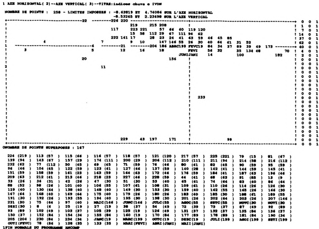
FIGURA 12- REPRESENTAÇÃO DOS INDIVÍDUOS (ESTAÇÕES PLUVIOMÉTRICAS) E VARIÁVEIS (CHUVA E IVDN) NO PLANO DEFINIDO PELA SEGUNDA COMPONENTE PRINCIPAL (EIXO HORIZONTAL) E PELA TERCEIRA COMPONENTE PRINCIPAL (EIXO VERTICAL)
