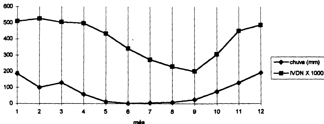
Figura 16-Comparação Gráfica dos Valores Originais Médios Mensais de Chuva e IVDN para o GRUPO DOIS
