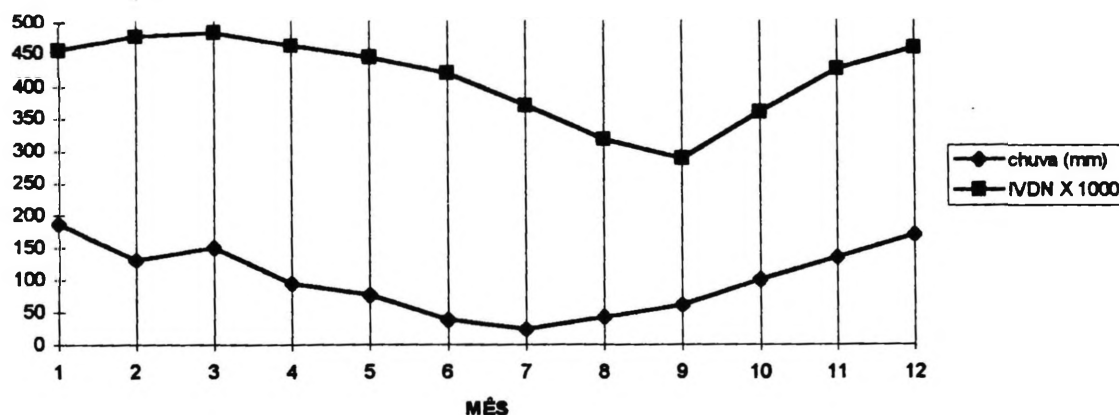
Figura 15- Comparação Gráfica dos Valores Originais Médios Mensais de Chuva e IVDN para o GRUPO UM
