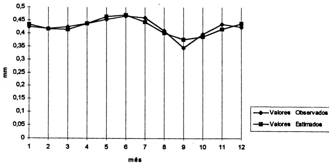
Figura48 Comparação Gráfica dos Valores Observados e Estimados de IVDN para o GRUPO SETE
