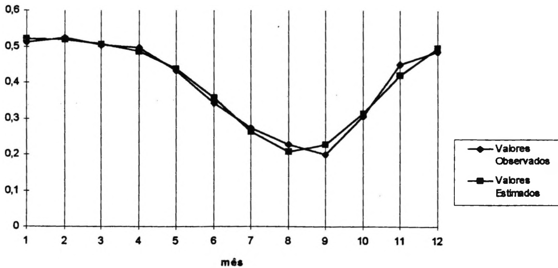
Figura 38 Comparação Gráfica dos Valores Observados e Estimados de IVDN para o GRUPO DOIS
