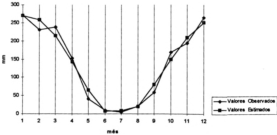
Figura 49 Comparação Gráfica dos Valores Observados e Estimados de Chuva para o GRUPO OITO
