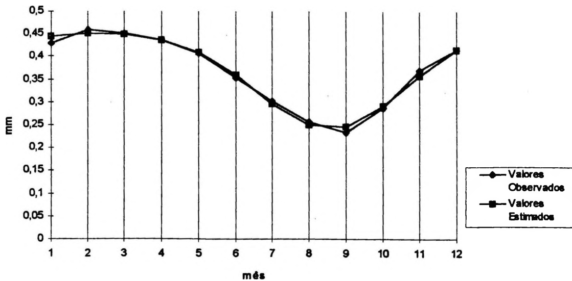
Figura40 Comparação Gráfica dos Valores Observados e Estimados de IVDN para o GRUPO TRÊS
