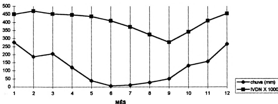
Figura 20- Comparação Gráfica dos Valores Originais Médios Mensais de Chuva e IVDN do GRUPO SEIS
