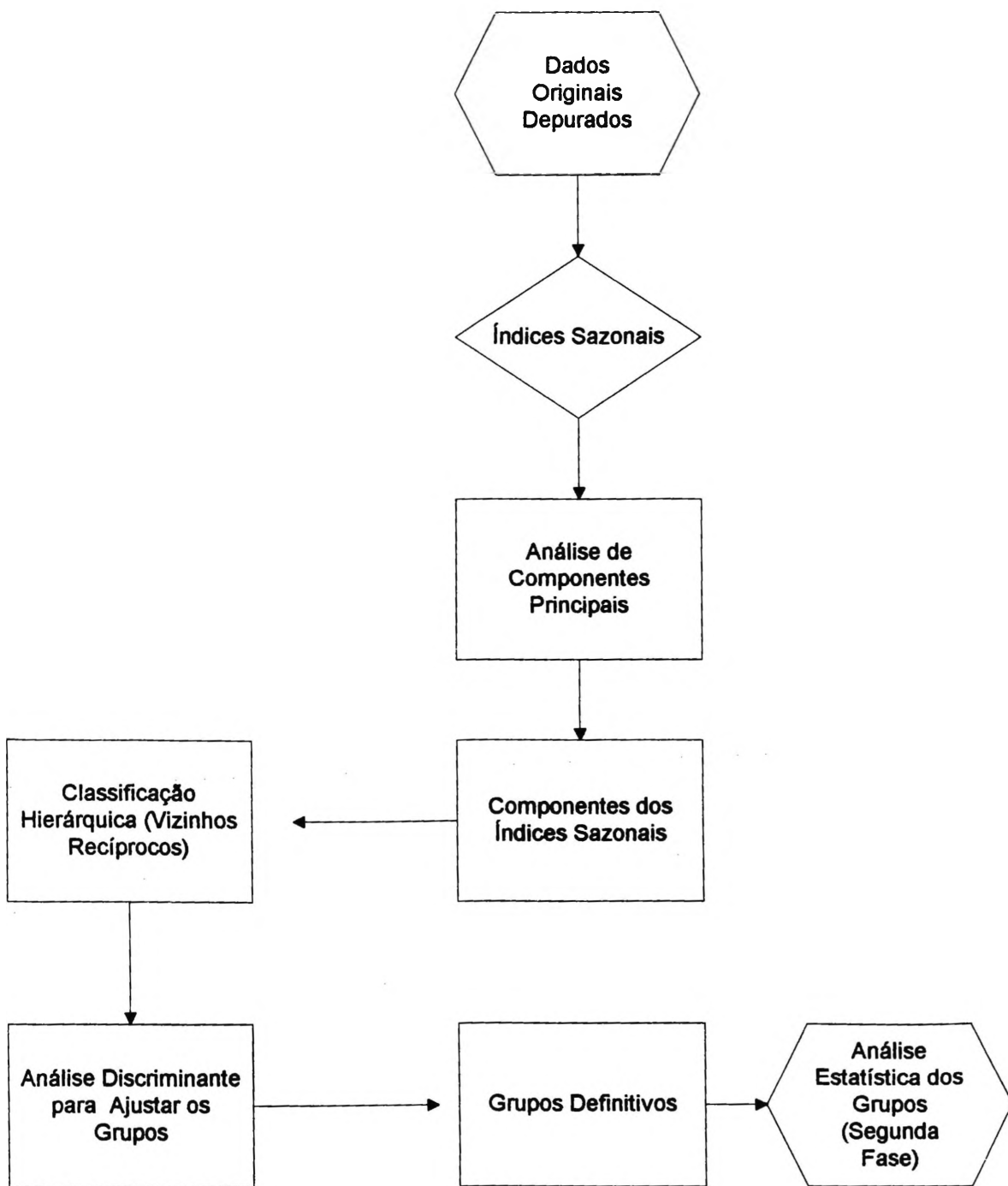
FIGURA 7-FLUXOGRAMA DOS MÉTODOS ESTATÍSTICOS UTILIZADOS PARA DETERMINAÇÃO DOS GRUPOS (ESTAÇÃO x IVDN) DE COMPORTAMENTO SIMILARES (PRIMEIRA FASE)
