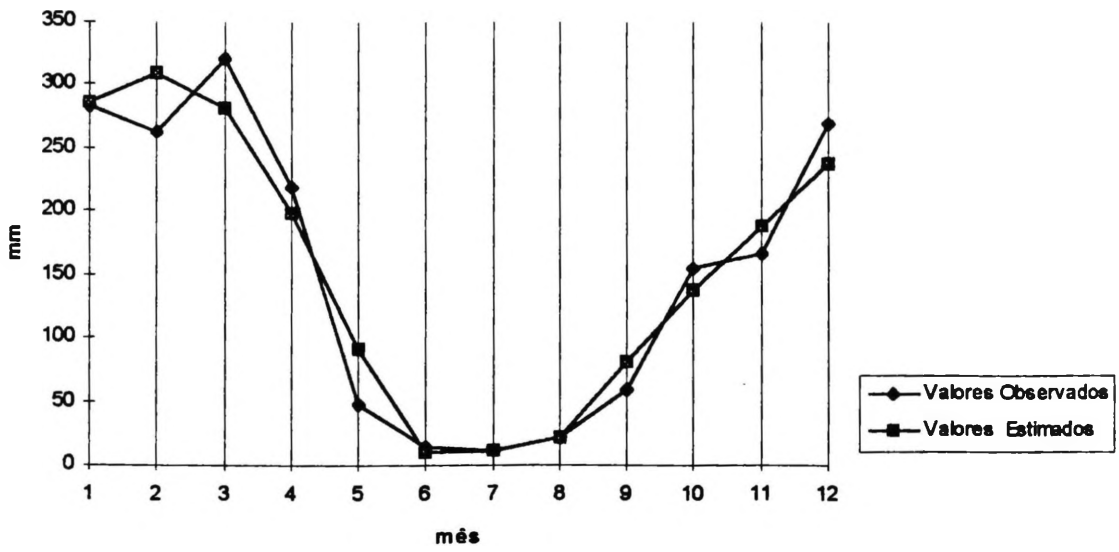
Figura 51 Comparação Gráfica dos Valores Observados e Estimados de Chuva para o GRUPO NOVE
