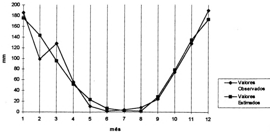
Figura 37 Comparação Gráfica dos Valores Observados e Estimados de Chuva para o GRUPO DOIS
