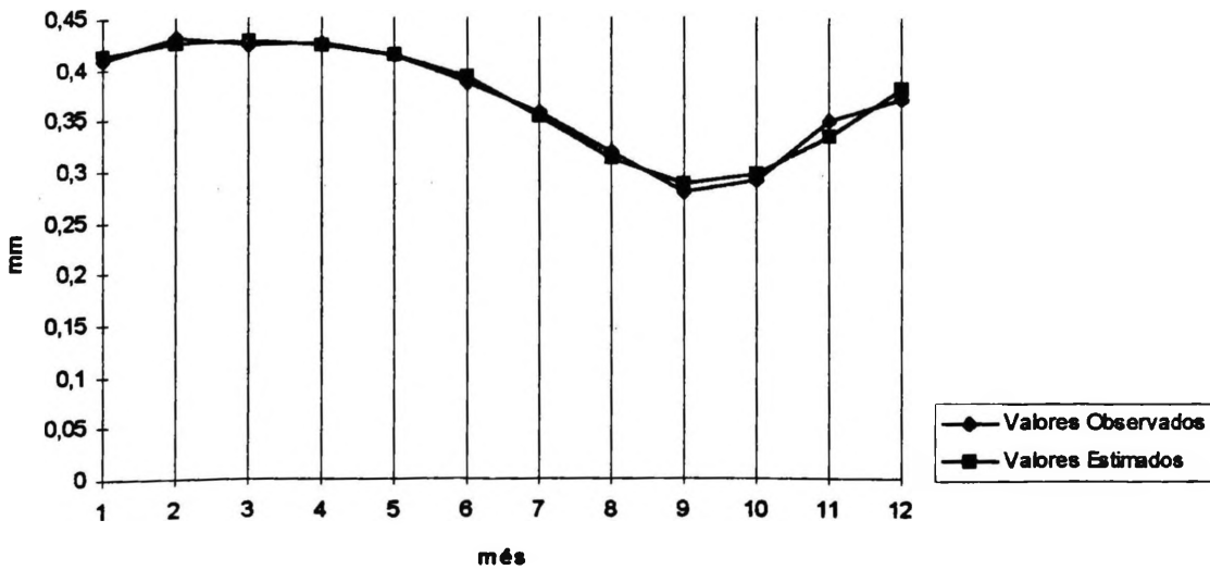
Figura 4.2 Comparação Gráfica dos Valores Observados e Estimados de IVDN para o GRUPO QUATRO
