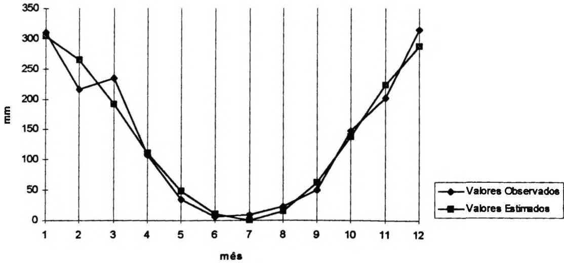
Figura43 Comparação Gráfica dos Valores Observados e Estimados de Chuva para o GRUPO CINCO
