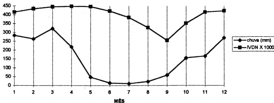
Figura 23- Comparação Gráfica dos Valores Originais Médios Mensais de Chuva e IVDN do GRUPO NOVE
