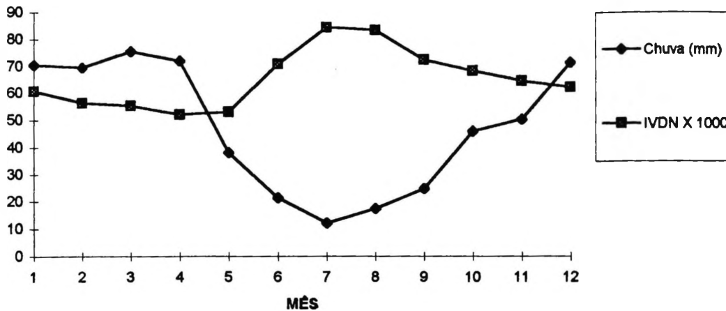
Figura 32- Demonstração Gráfica do Desvio Padrão Geral Mensal de Chuva e IVDN para os Dez Grupos
