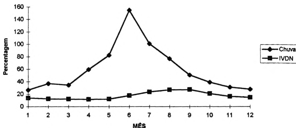
Figura 31- Demonstração Gráfica dos Coeficientes de Variação Mensais Gerais entre Chuva e IVDN
