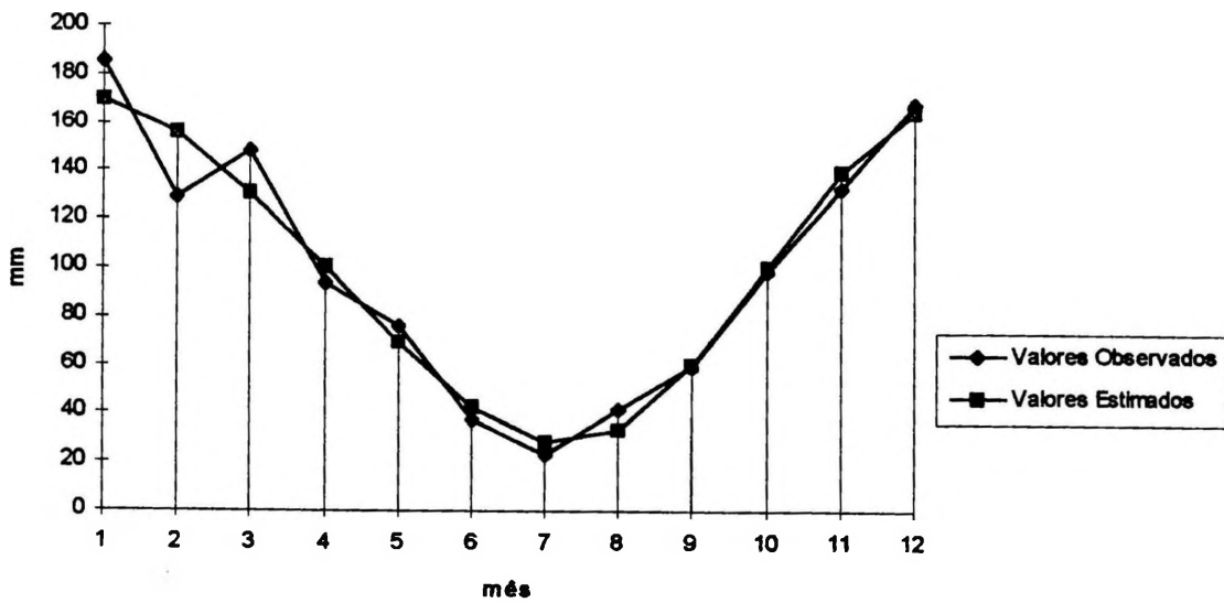
Figura 35 Comparação Gráfica dos Valores Observados e Estimados de Chuva para o GRUPO UM
