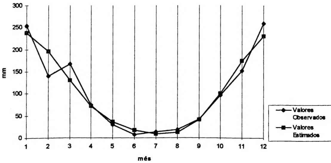
Figura 4.1 Comparação Gráfica dos Valores Observados e Estimados de Chuva para o GRUPO QUATRO
