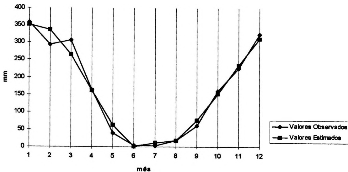
Figura47 Comparação Gráfica dos Valores Observados e Estimados de Chuva para o GRUPO SETE
