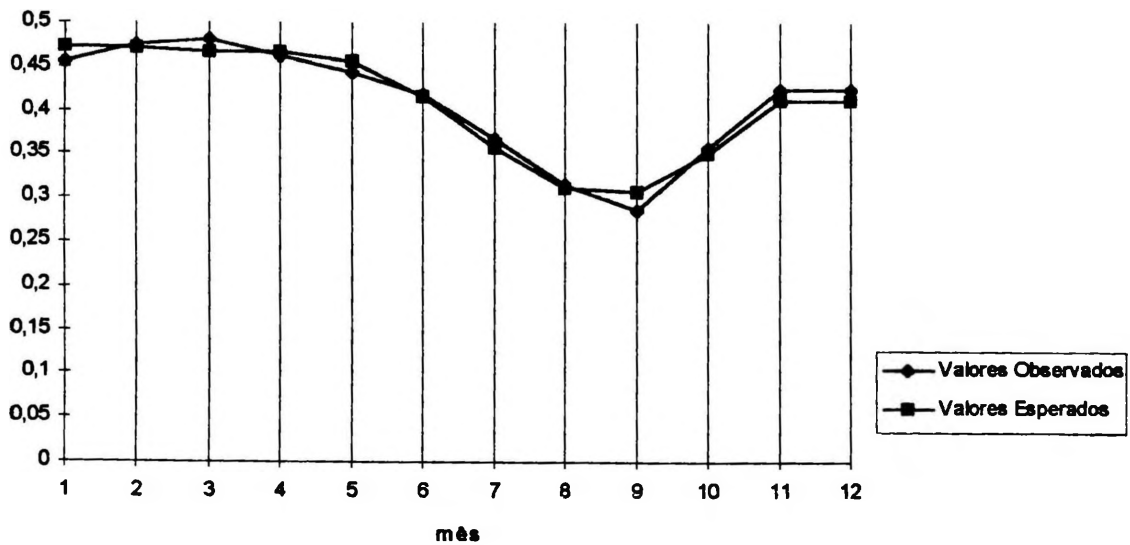
Figura 36 Comparação Gráfica dos Valores Observados e Estimados de IVDN para o GRUPO UM
