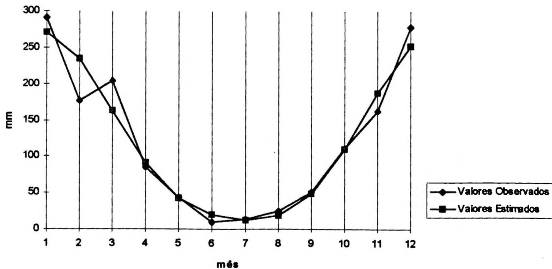
Figura39 Comparação Gráfica dos Valores Observados e Estimados de Chuva para o GRUPO TRÊS
