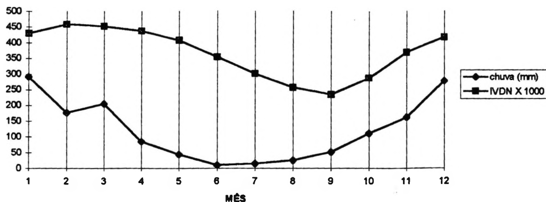
Figura 17- Comparação Gráfica dos Valores Originais Médios Mensais de Chuva e IVDN para o GRUPO TRÊS
