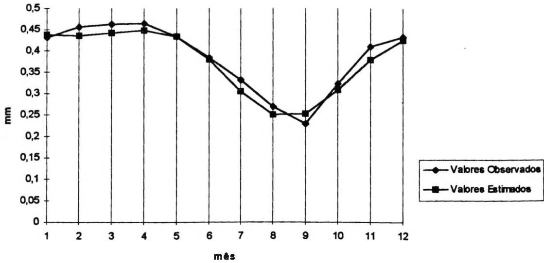
Figura44 Comparação Gráfica dos Valores Observados e Estimados de IVDN para o GRUPO CINCO
