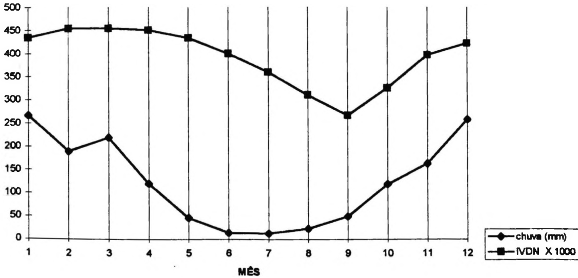
Figura 27- Comparação Gráfica dos Valores Originais Médios Mensais Gerais de Chuva e IVDN para as 234 Estações Pluviométricas
