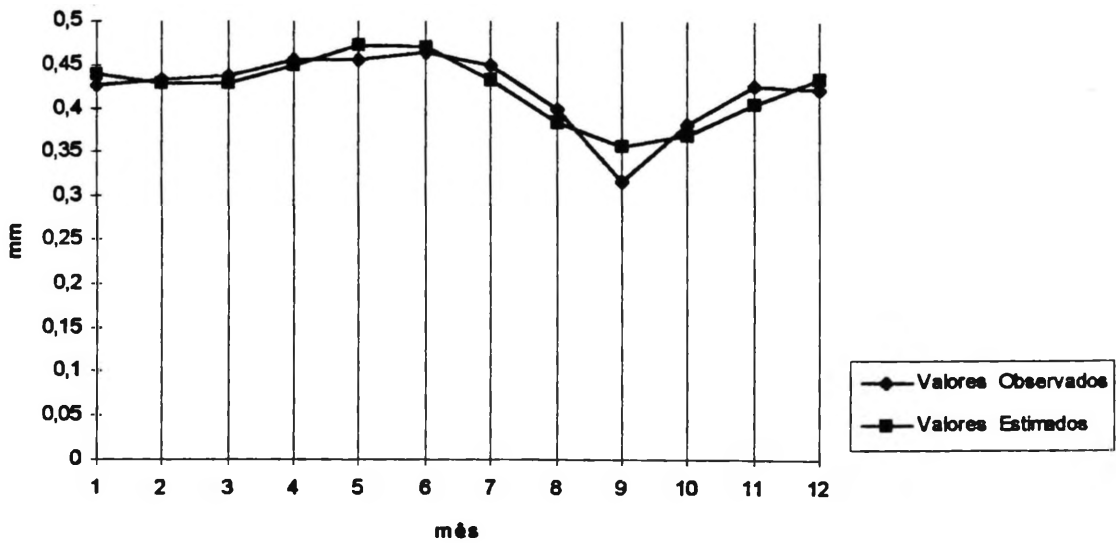
Figura 50 Comparação Gráfica dos Valores Observados e Estimados de IVDN para o GRUPO OITO
