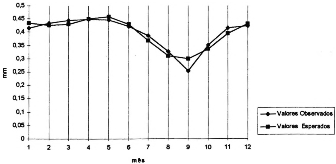
Figura 52 Comparação Gráfica dos Valores Observados e Estimados de IVDN para o GRUPO NOVE
