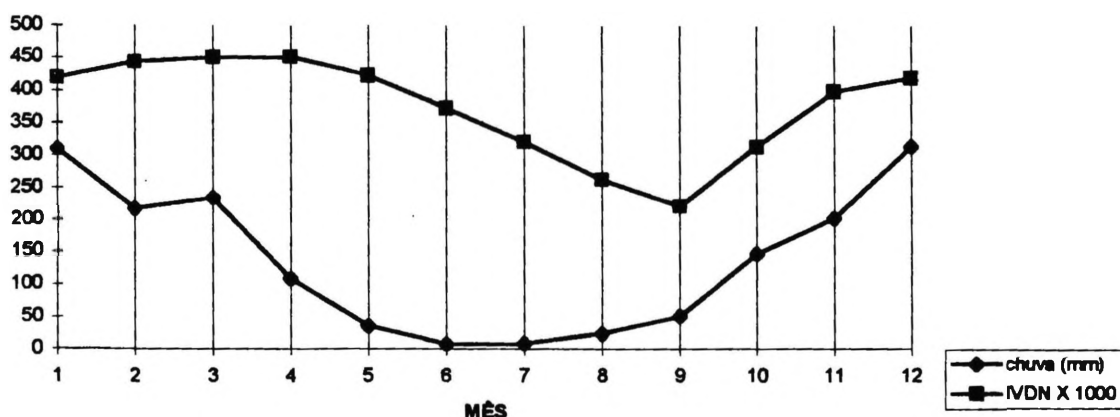
Figura 19- Comparação Gráfica dos Valores Originais Médios Mensais de Chuva e IVDN para o GRUPO CINCO
