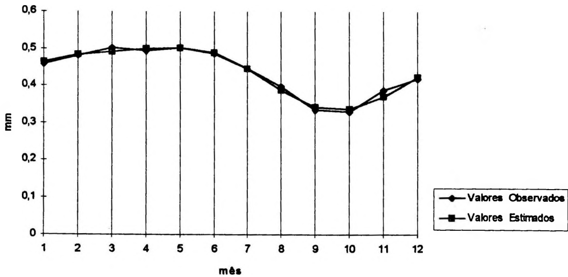
Figura54 Comparação Gráfica dos Valores Observados e Estimados de IVDN para o GRUPO DEZ
