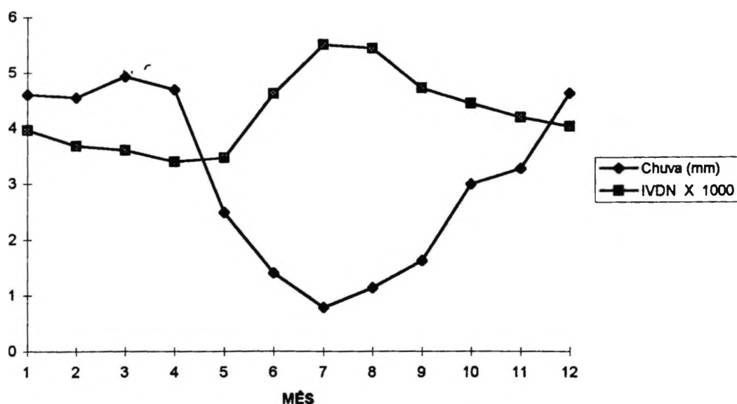
Figura 33 Demonstração Gráfica do Erro Padrão Geral Mensal de Chuva e IVDN para os Dez Grupos
