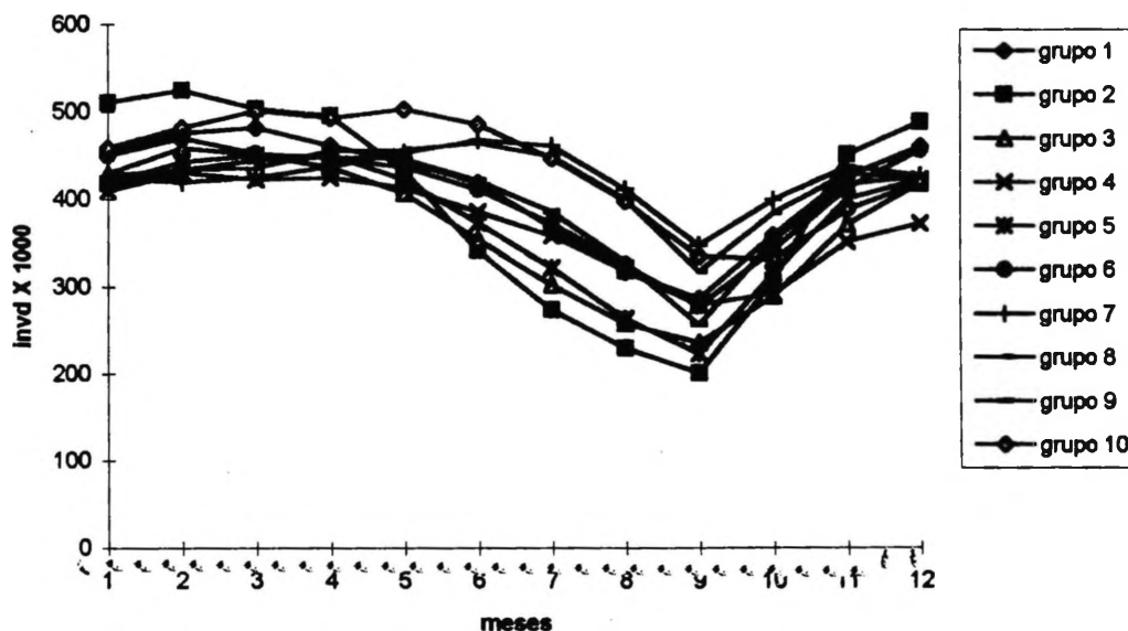
Figura26 Demonstração Gráfica da Distribuição Multitemporal do IVDN para cada um dos Dez Grupos
