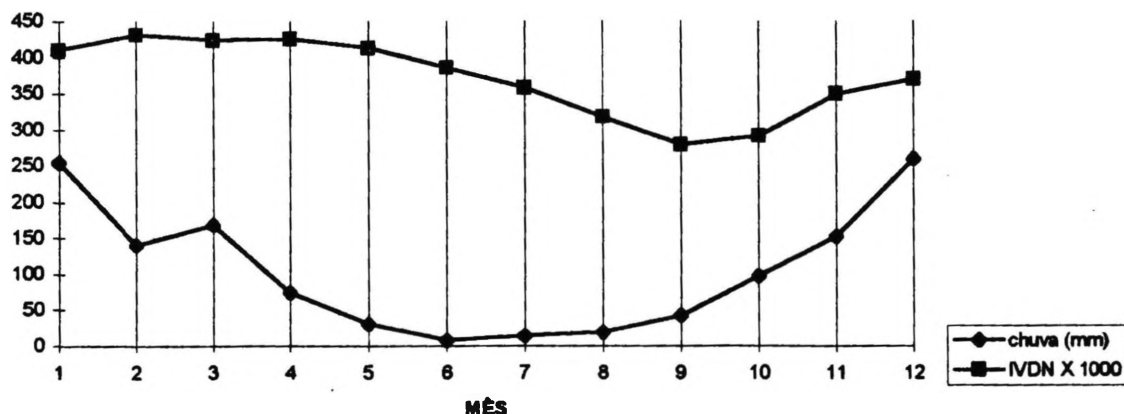
Figura 18- Comparação Gráfica dos Valores Originais Médios Mensais de Chuva e IVDN para o GRUPO QUATRO
