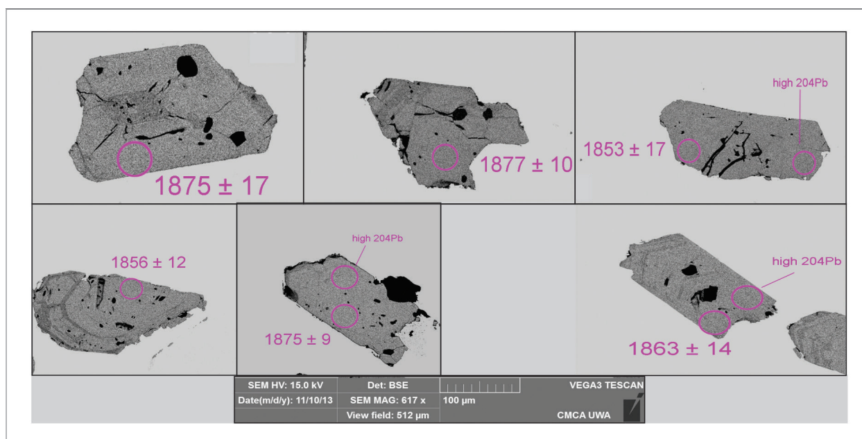
Figura 11. Imagem retro-espalhado de microscopia eletrônica de varredura de cristais de zircão do biotita monzogranito (FR29) mostrando sua morfologia e os locais de aplicação do feixe de O_2 .
