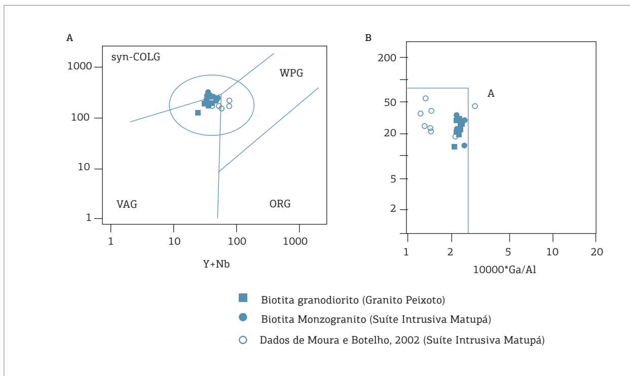
Figura 10. Diagramas de discriminação tectônica. (A) Rb versus Y+Nb (Pearce et al. 1996) e (B) 10000*Ga/Al versus Y (Whalen et al. 1987).
