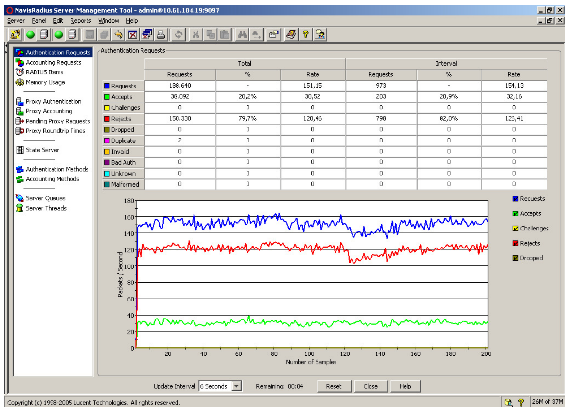
Figura 5.16: Requisições de autenticação recebidas por um servidor RADIUS, durante a implementação do recurso lista negra dinâmica.
