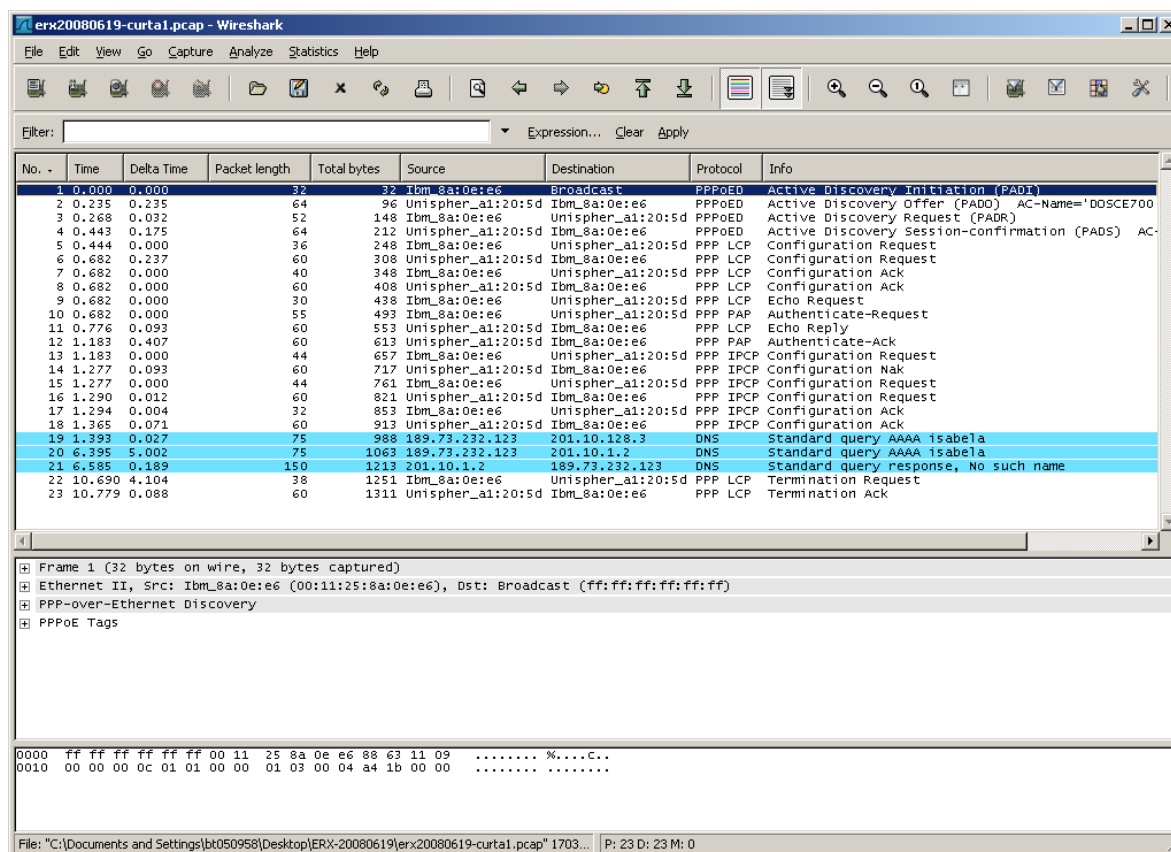
Figura 5.5: Captura de tráfego para uma conexão PPPoE com o NAS Juniper ERX 1440
