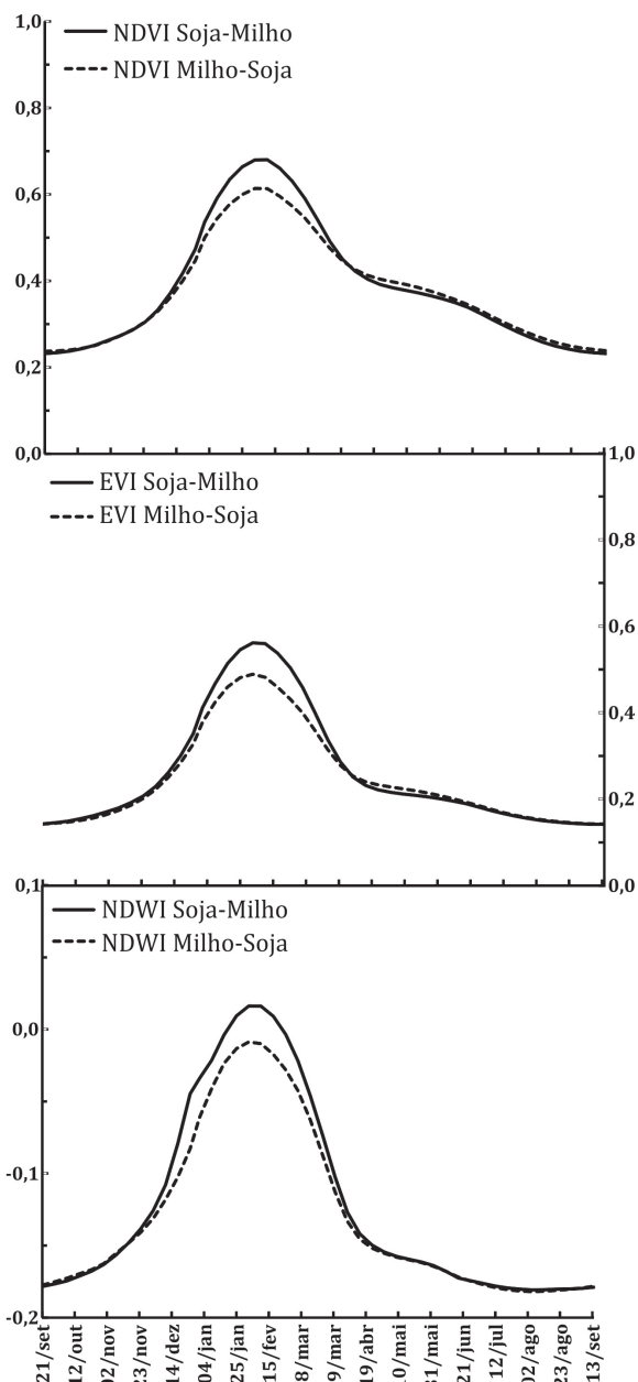
Fig. 8—Comportamento temporal médio dos índices de vegetação NDVI, EVI e NDWI referentes às sucessões soja-milho e milho-soja.
