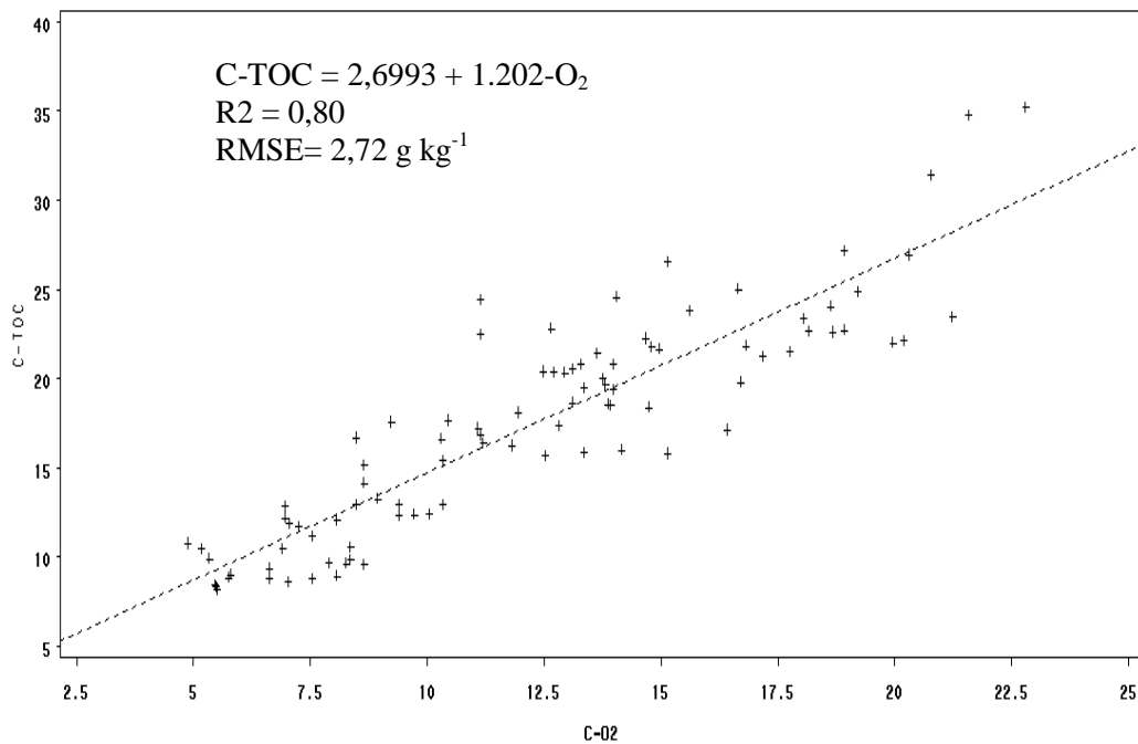
Figura 9. Regressão linear entre os teores de C orgânico total ( \text{g kg}^{-1} ) por combustão a seco (C-TOC) e oxidação via úmida sem aquecimento externo (C-O 2 ) em um Latossolo Vermelho argiloso no Cerrado de 0-100 cm. ( p < 0.001 ; n = 48 ).
