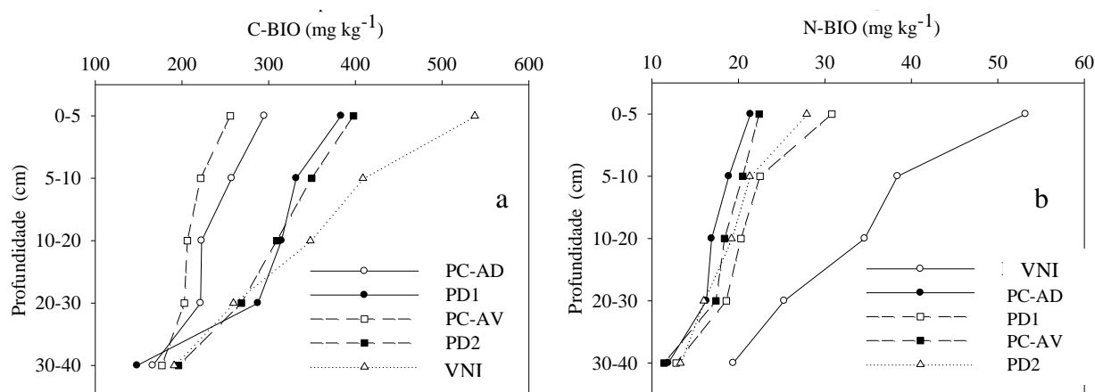
Figura 16. Distribuição da biomassa microbiana no perfil de 0-40 cm de um Latossolo Vermelho argiloso sob diferentes sistemas de manejo no Cerrado.
