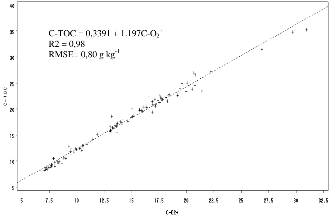
Figura 8. Regressão linear entre os teores de C orgânico total ( \text{g kg}^{-1} ) por combustão a seco (C-TOC) e oxidação via úmida com aquecimento (C-O 2 + ) em um Latossolo Vermelho argiloso no Cerrado de 0-100 cm. ( p < 0.0001 ; n = 48 ).
