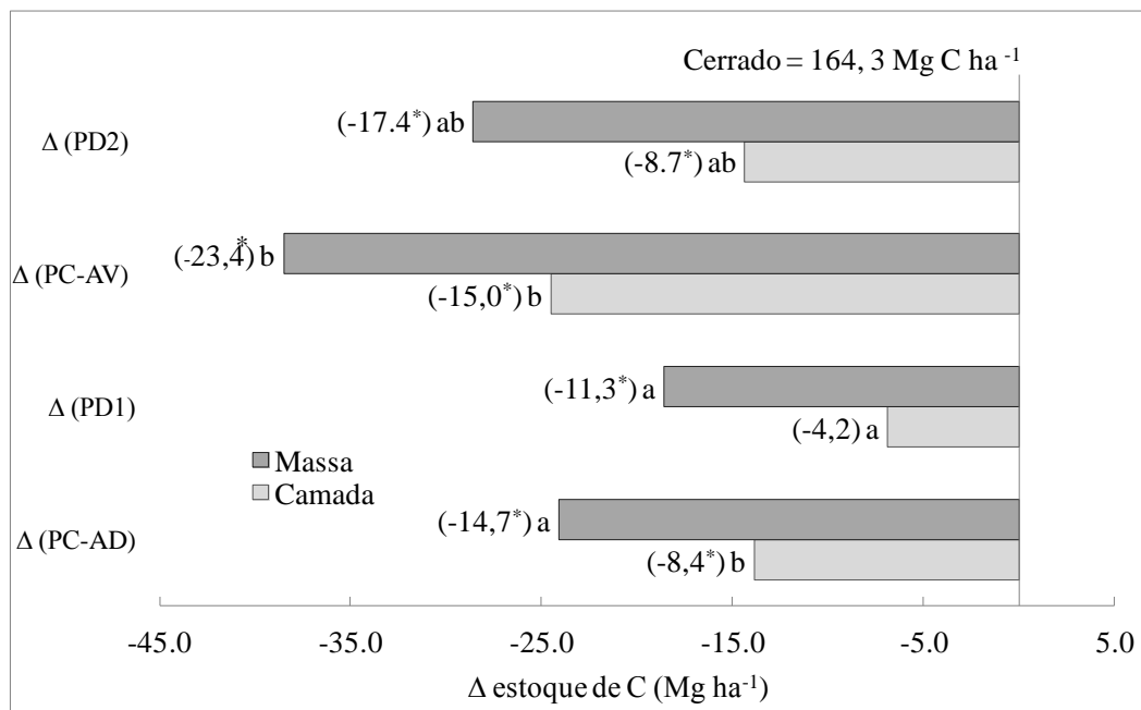
Figura 7. Diferenças absolutas e relativas de estoque de carbono do solo no intervalo de 0-100 cm de profundidade. *significativo pelo teste t ( p < 0,05 ) pareado entre: (PD2) PD2 e VN1; (PC-AV) PC-AV e VN1; (PD1) PD1 e VN1; (PC-AV) PC-AV e VN1. Médias seguidas da mesma letra na Camada ou na Massa indicam que não há diferenças significativas entre si pelo teste t ( p < 0,05 ) entre os sistemas cultivados. Perdas são indicadas pelo sinal negativo (-). Valores em parênteses representam as mesmas diferenças expressas em porcentagem. Camada : estoques de C calculados pela camada equivalente, sem correção pela massa de solo equivalente ao sistema natural de referência [VN1]; Massa : estoques de C corrigidos pela massa equivalente de solo equivalente ao sistema natural de referência [VN1].
